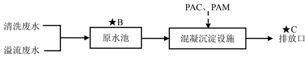
图 3.4 废水处理工艺流程图
