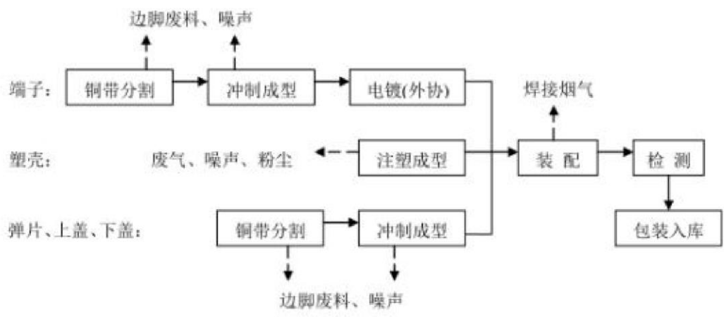
图 3.3 工艺流程图
