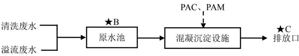
图 3.4 废水处理工艺流程图
