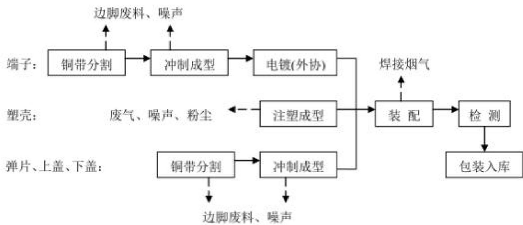
图 3.3 工艺流程图
